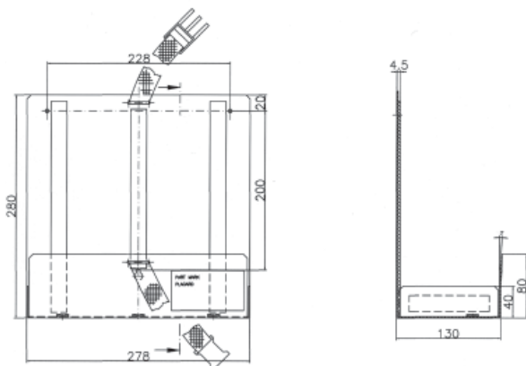
PNR 6240-37 • Bracket
