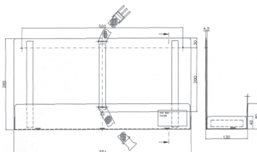
PNR 6240-01-001 • Bracket
